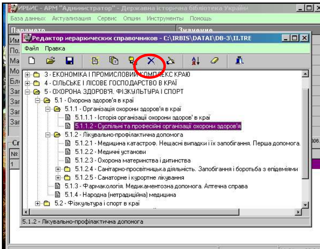
Мал. 14. Вилучення непотрібного елемента – буде вилучений виділений пункт
